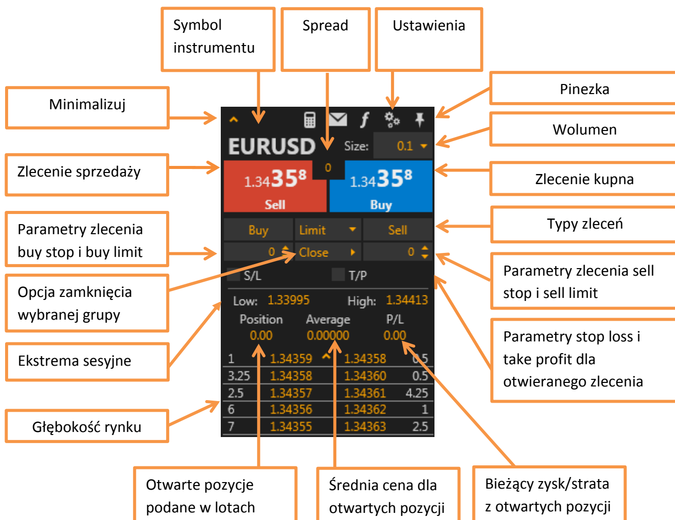
Rysunek 2: Główny interfejs.
