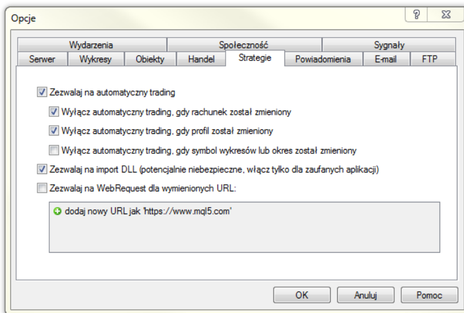
Rysunek 1: Poprawnie skonfigurowane opcje strategii.
